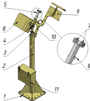
Рисунок 2. Схема изделия
