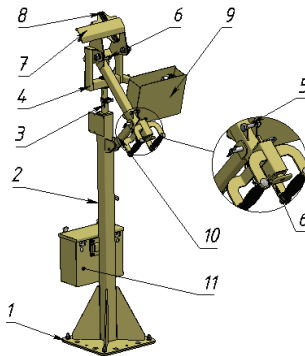
Рисунок 2. Схема изделия
